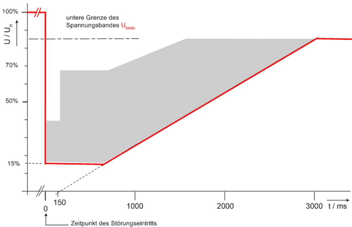
Bild 3-2 Verbleiben von Erzeugungsanlagen mit geringem Kurzschlussstromanteil am Netz bei Anschlusspunkt nahen Fehlern
